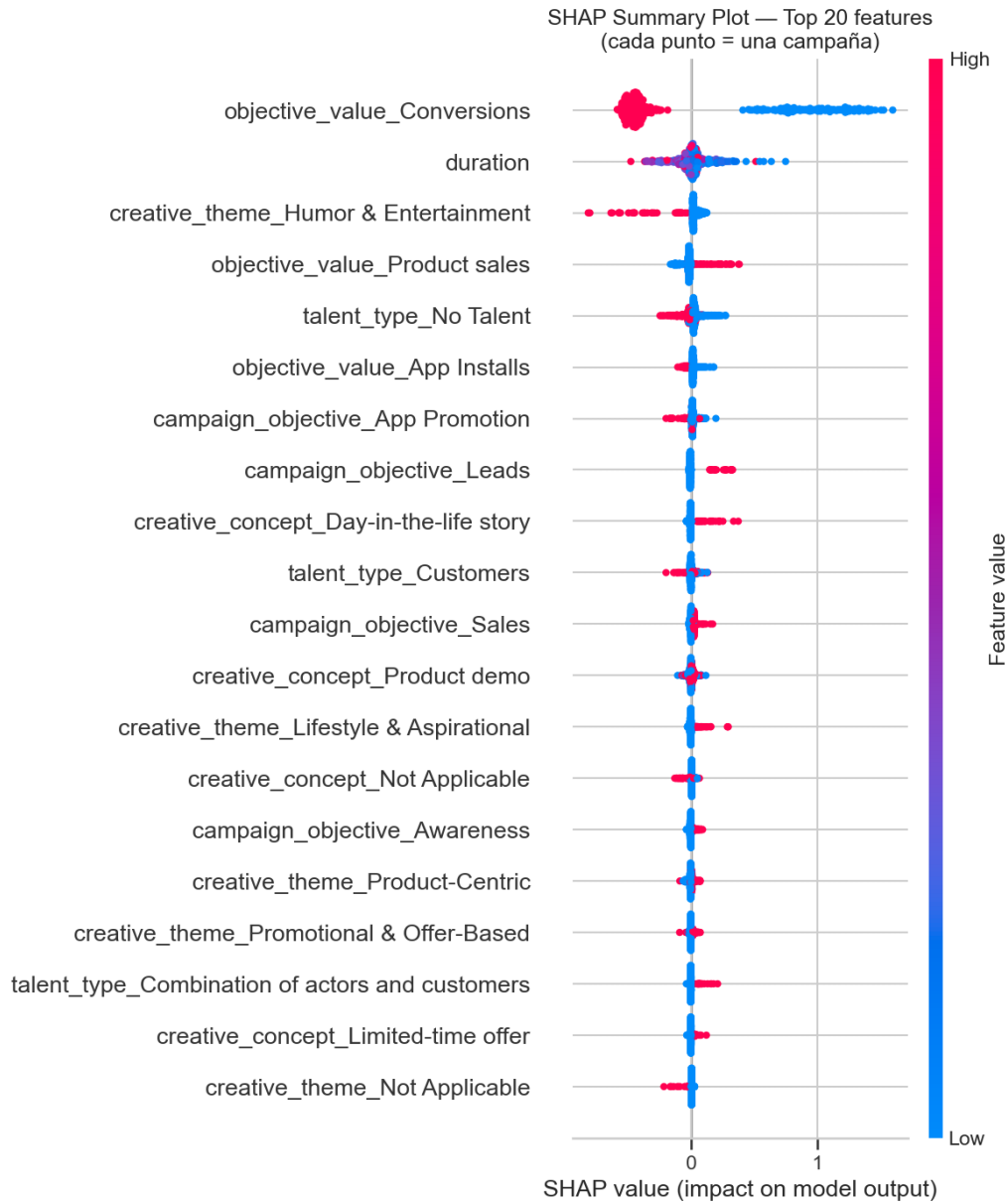
Figura 4.4: SHAP beeswarm plot : las 20 variables con mayor importancia promedio |\text{SHAP}| . Cada punto representa una observación. El color indica el valor de la variable (rojo = alto, azul = bajo); la posición horizontal indica el impacto en la predicción del modelo.
