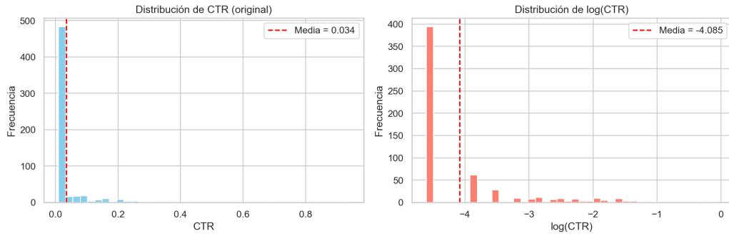
Figura 4.1: Distribución del CTR: escala original (izquierda) y transformación logarítmica (derecha). La asimetría pronunciada de la escala original justifica el uso de \log(\text{CTR}) como variable dependiente.
