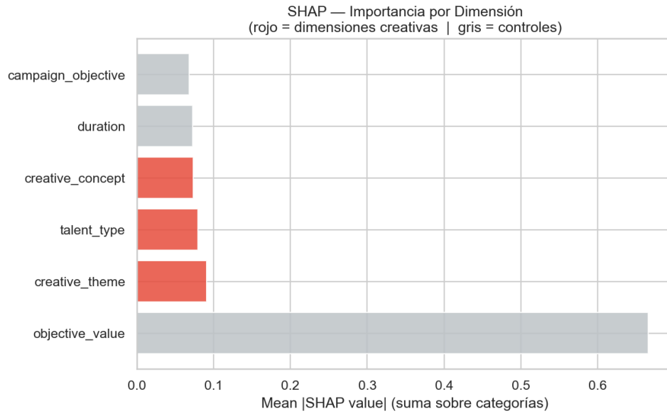
Figura 4.5: Importancia SHAP media ( |\text{SHAP}| ) agregada por dimensión creativa. Las barras representan la contribución promedio de cada dimensión a las predicciones del modelo Random Forest.
