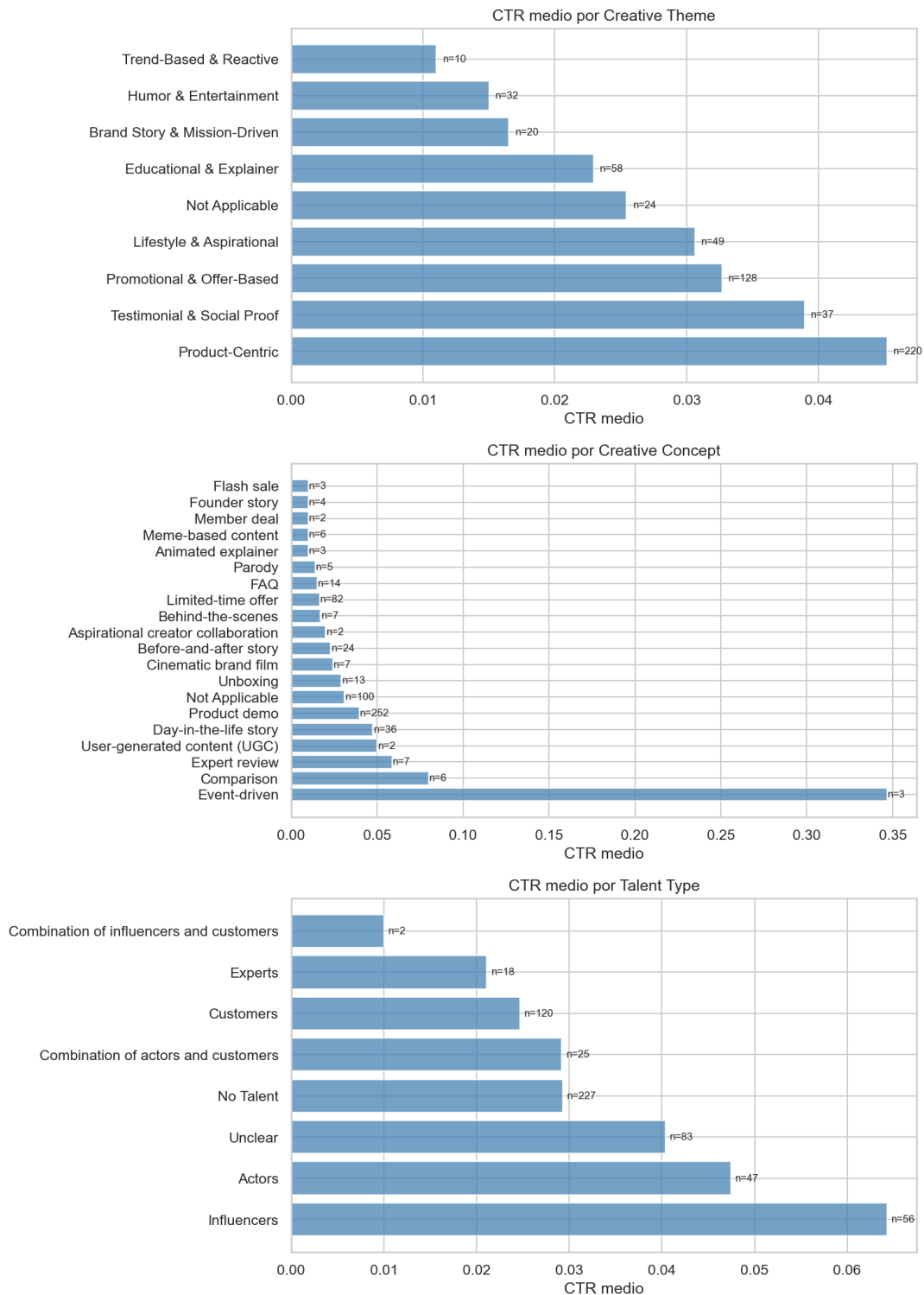
Figura 4.2: CTR medio por categoría para las tres dimensiones creativas analizadas. Las barras representan el CTR promedio por grupo; el tamaño de muestra por categoría varía considerablemente.
