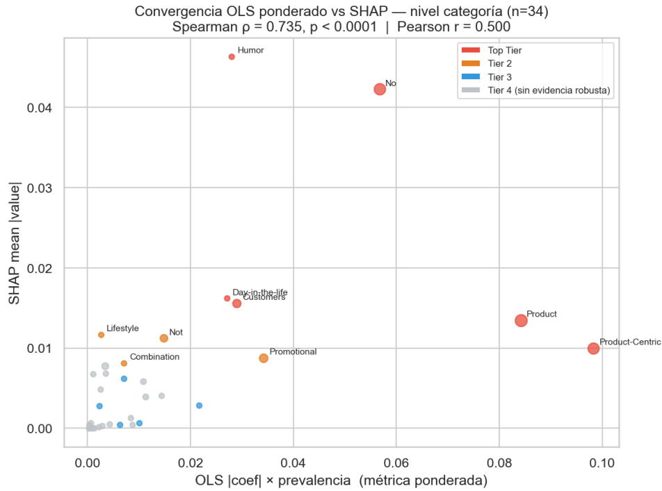
Figura 4.6: Convergencia entre OLS (coeficiente ponderado por prevalencia) y SHAP ( |\text{SHAP}| promedio) a nivel de categoría individual ( n = 34 ). La correlación de Spearman es \rho = 0,74 ( p < 0,001 ).
